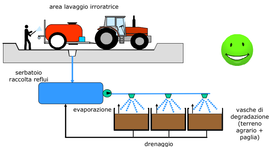
Fig. 91 - Raccolta delle acque reflue del lavaggio e loro biodegradazione (biobac ® ). Il contenuto delle vasche di degradazione viene monitorato e periodicamente arieggiato e rivoltato e deve essere sostituito ogni circa 5 anni. Tale terreno esausto può poi essere distribuito in campo
