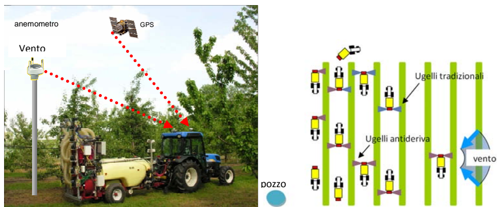
Fig. 167 – Irrigatrice con sensori per l'adattamento della distribuzione alle condizioni ambientali
